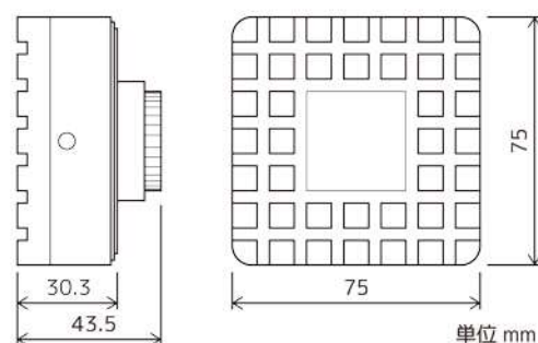
◎ カメラ寸法図
